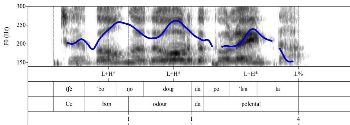
Fig. 29.13. Spectrogram, curve di F0 (in blu) e anotazion prosodiche de esclamazion "Ce bon odour da polenta!" pronunciade di une persone che e fevele furlan ocidentâl (Tesis).
