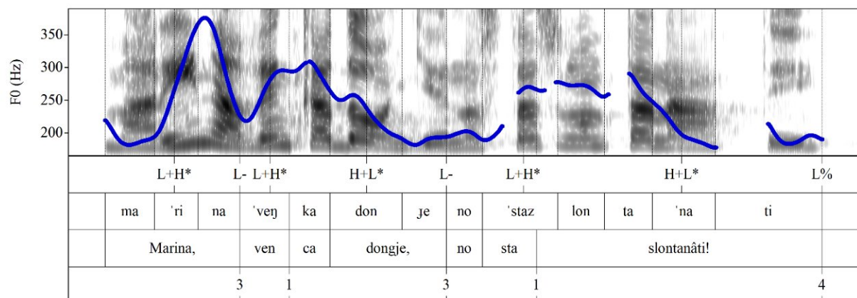
Fig. 29.14. Spetrogram, curve di F0 (in blu) e anotazion prosodiche dal ordin “Marina, ven ca dongje, no sta slontanâti!” pronunciade di une persone che e fevele furlan centrâl (Remanzâs).
