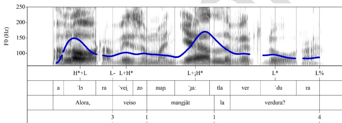
Fig. 29.10. Spectrogram, curve di F0 (in blu) e anotazion prosodiche de domande totâl cuntun bias positîf “Alora, veiso mangjât la verdura?” pronunciade di une persone che e fevele cjargnel (Negrons).
