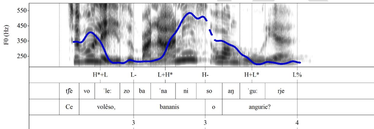
Fig. 29.5. Spectrogram, curve di F0 (in blu) e anotazion prosodiche de domande parziâl disiuntive “[Ce volêso,] bananis o angurie?” pronunciate di une persone che e fevele furlan centrâl (Remanzâs).
